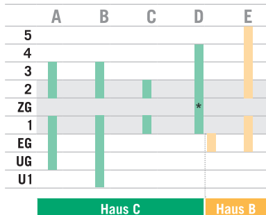
○ Aufzugs-/Etagenübersicht
